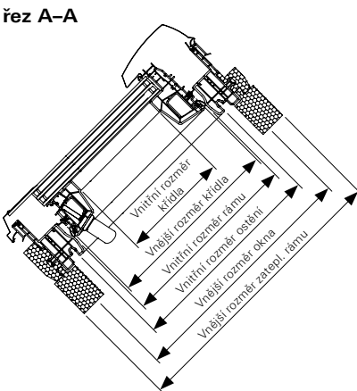
řez A–A
