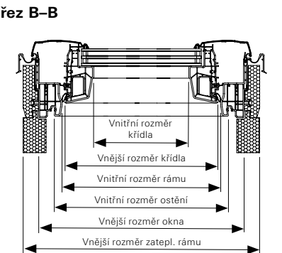
řez B–B
